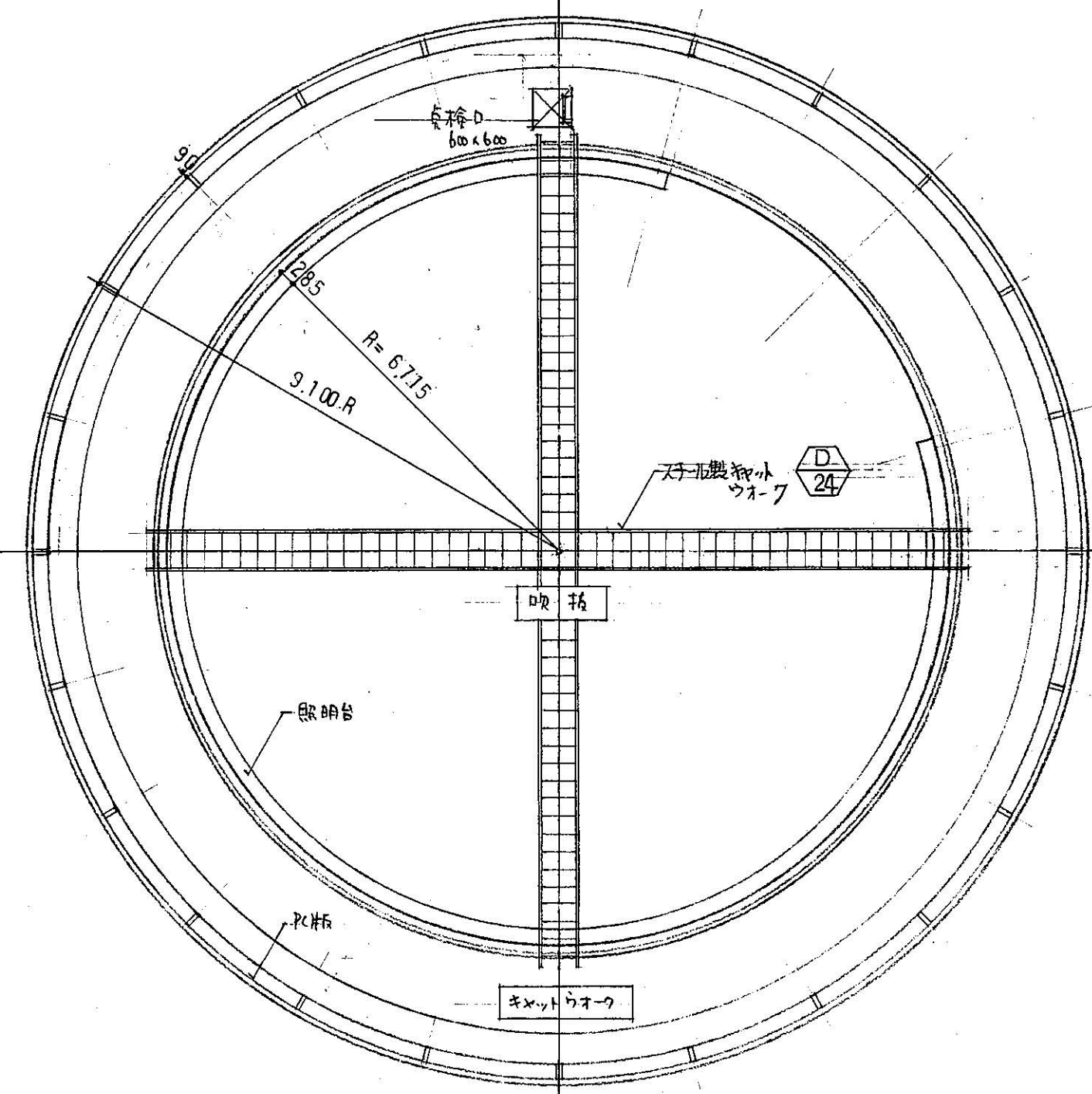
3F 平面図 1:100
