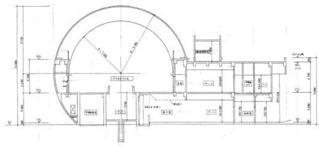
②-② 断面図 1:100
