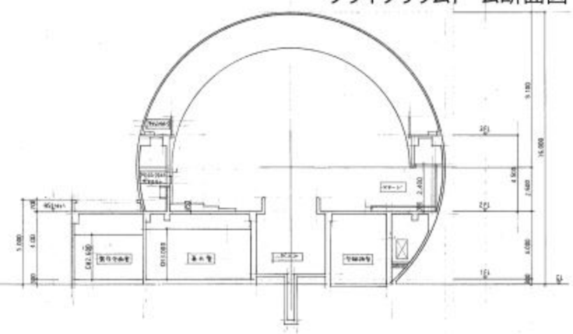
③-③ 断面図 1:100
