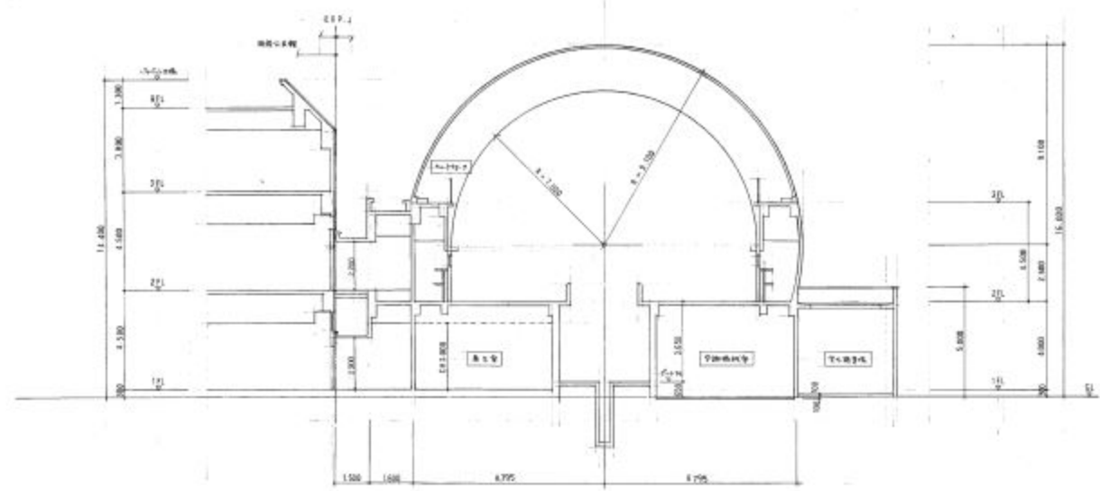
①-① 断面図 1:100
