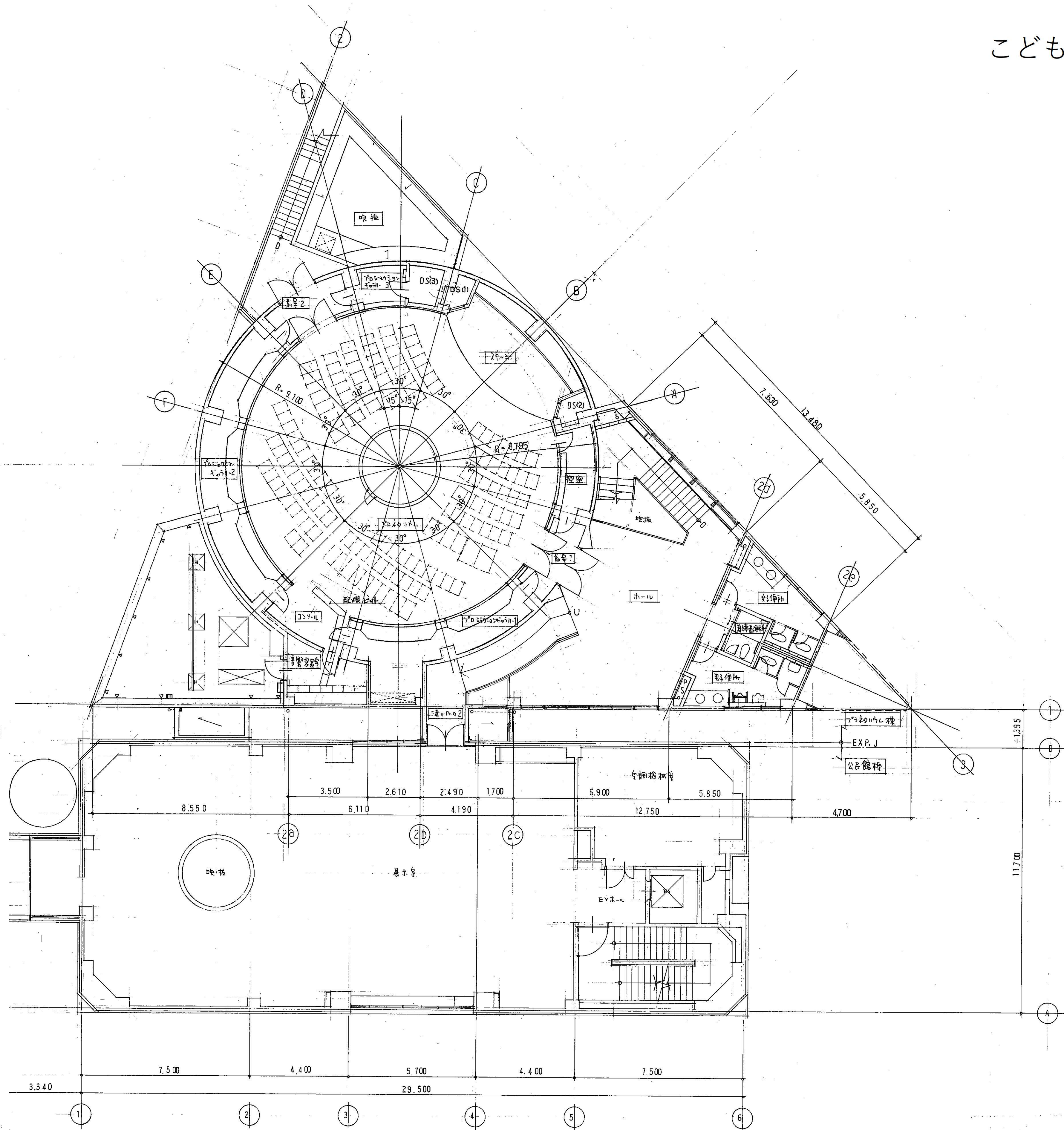
2F 平面図 1:100
