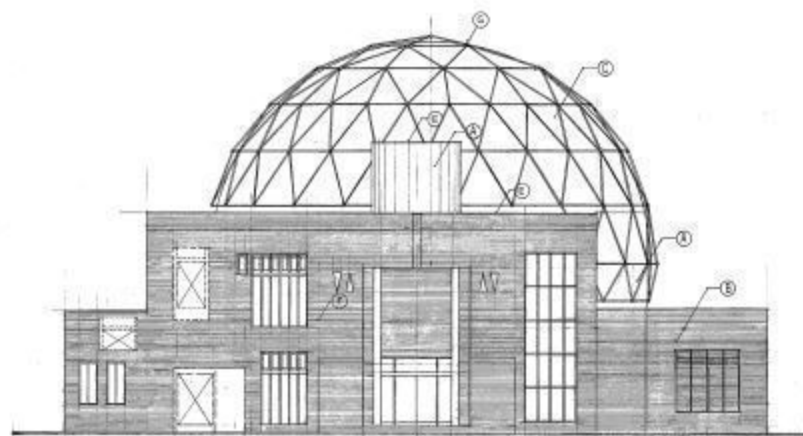
正面立面図 1:300
