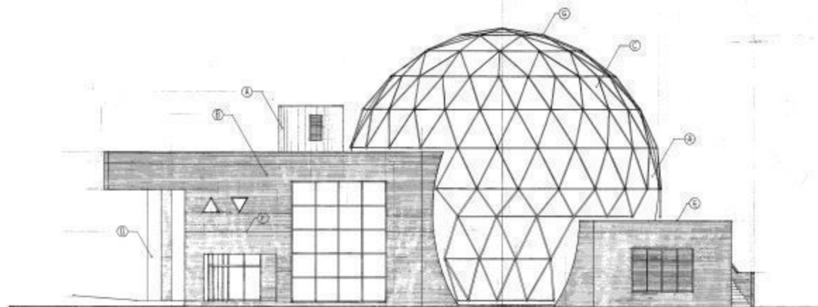
側面立面図 1:300
