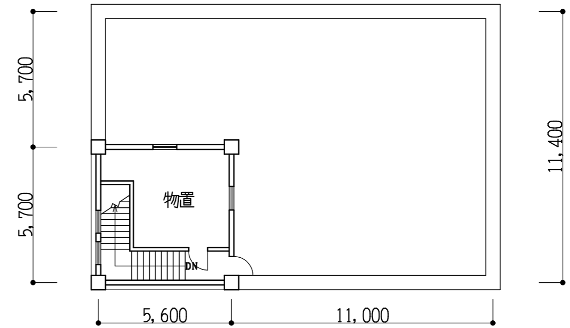
3階平面図 1/200
