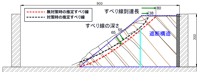
図-1 遠心載荷模型実験による遮断構造の制御効果（単位：mm）
