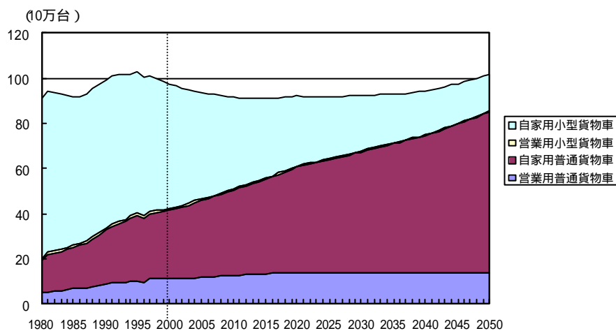
図 車種業態別貨物車保有台数(軽貨物車を除く)の推計結果
