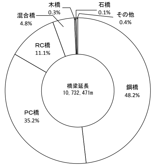
(ロ) 橋種別橋梁延長比率
