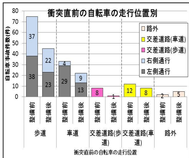
図4 衝突直前の自転車の走行位置別の事故件数比較
