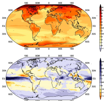
中学理科の教科書(東京書籍)で紹介された、気候モデルMIROCによる将来の気温(上)と降水量(下)の予測
