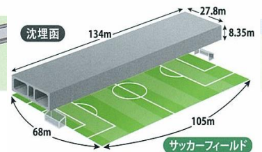
沈埋函の大きさ
