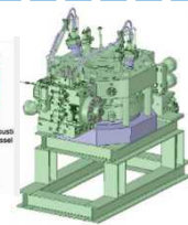
燃料噴射弁試験装置
