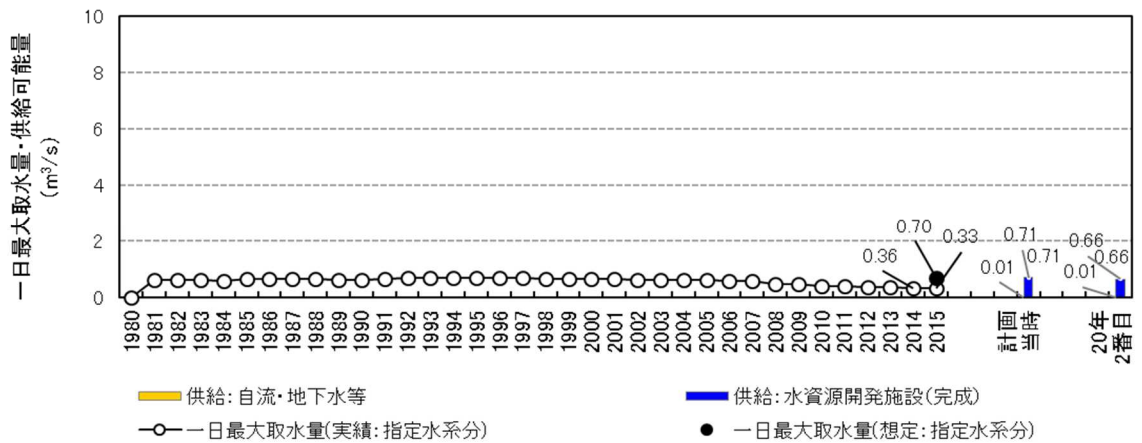
参考図表 5 9 工業用水 需要実績・想定と供給可能量の比較
