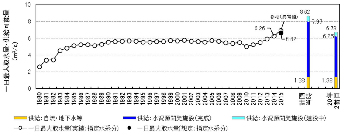
参考図表 5 7 都市用水 需要実績・想定と供給可能量の比較
