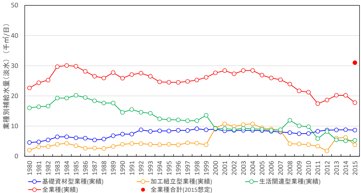
参考図表 5 1 業種別 補給水量(淡水)の推移
