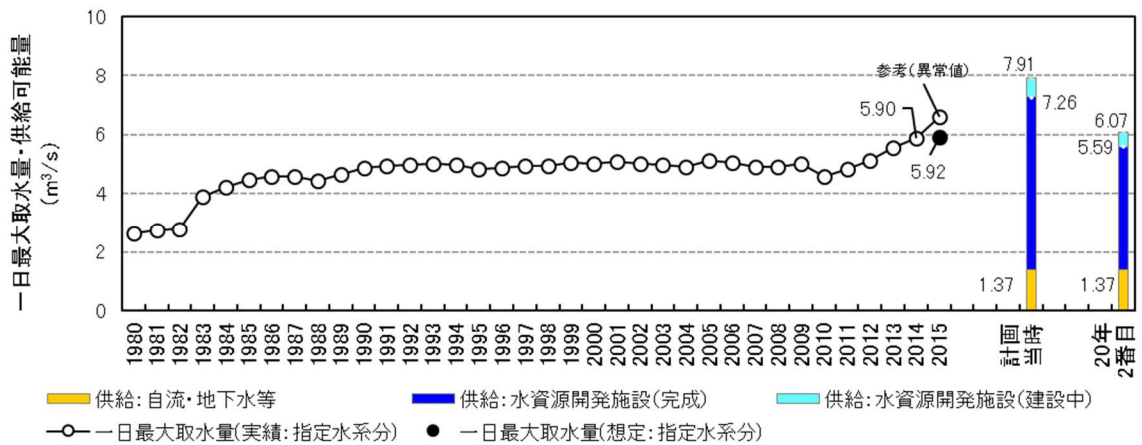
参考図表 5 8 水道用水 需要実績・想定と供給可能量の比較
