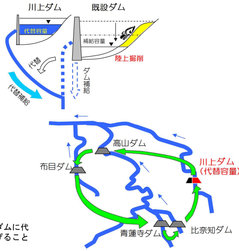
川上ダムによる代替補給イメージ図
