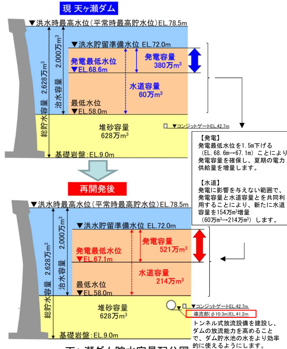
天ヶ瀬ダム貯水容量配分図
