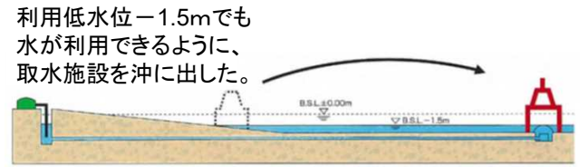
水位低下対策(取水口の沖出し)
