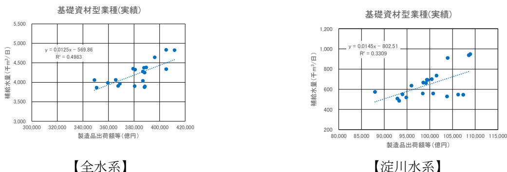
図 23 基礎資材型業種 補給水量と製造品出荷額等の相関
