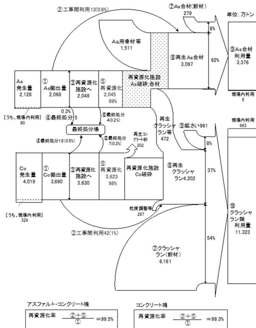
図 2-9 アスファルト・コンクリート塊、コンクリート塊のリサイクルフロー 19
