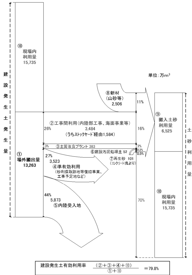
図 2-6 建設発生土のフロー 16
