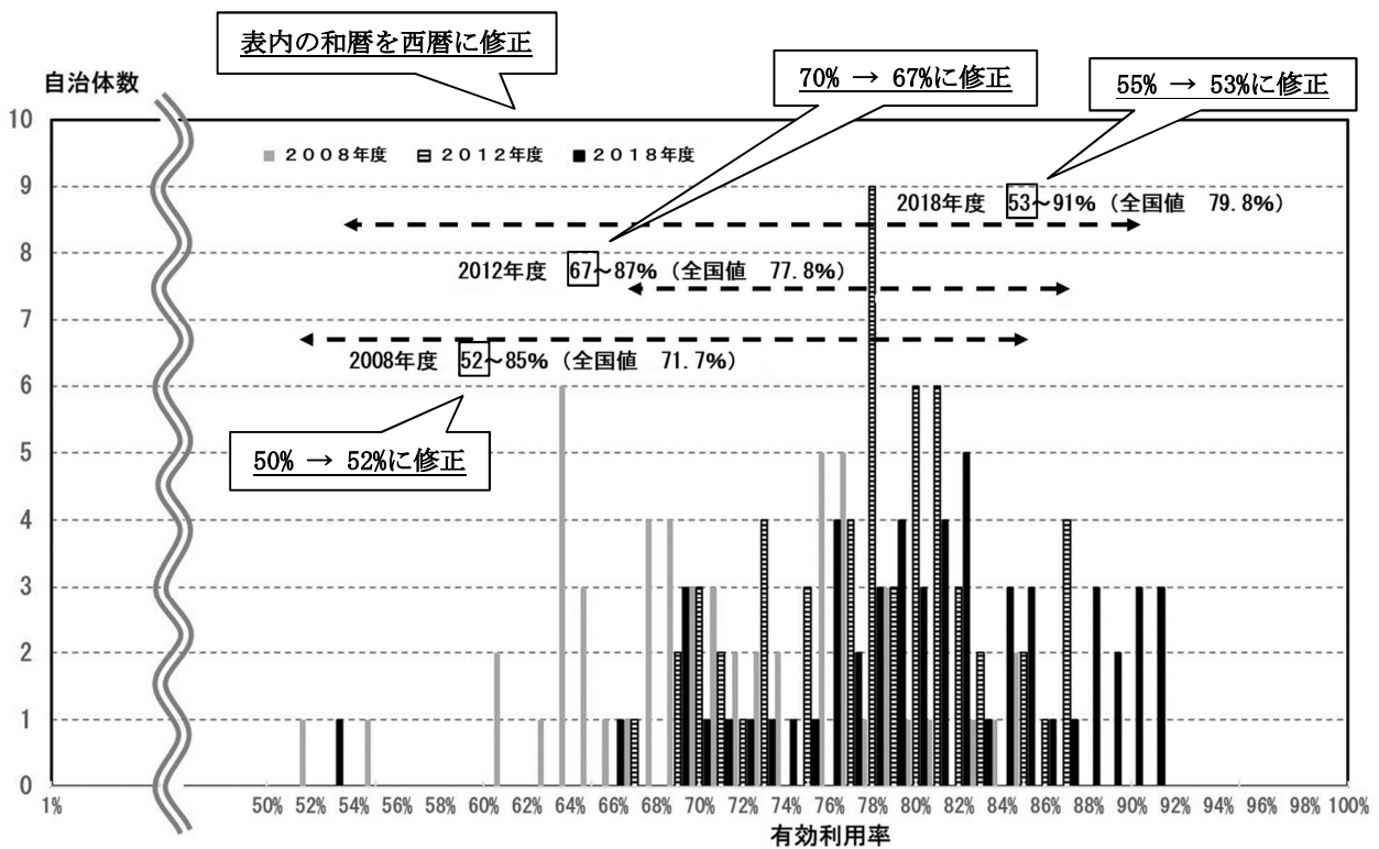
図 4-2 各自治体における建設発生土有効利用率 分布の推移
