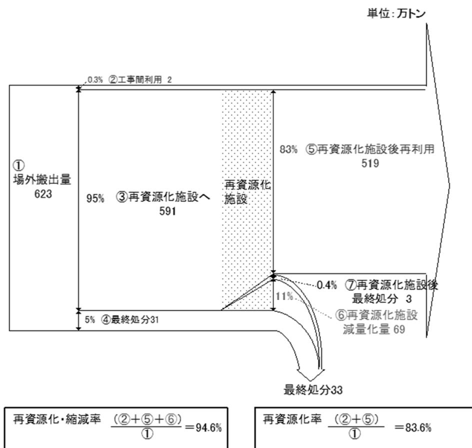
図 2-10 建設汚泥のリサイクルフロー 20
