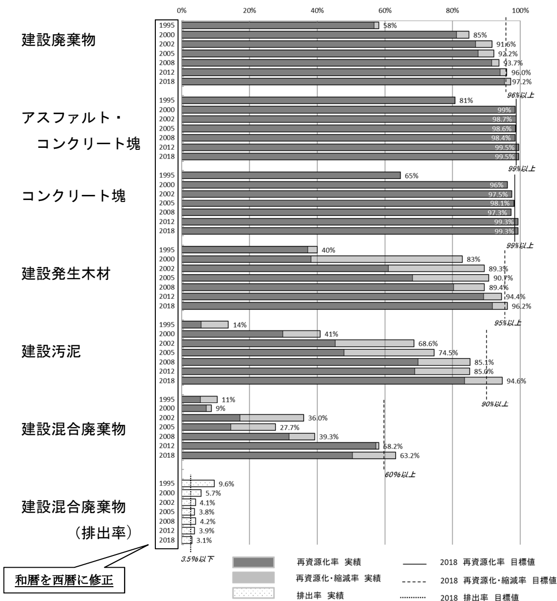
図2-1 品目別再資源化率等の推移
