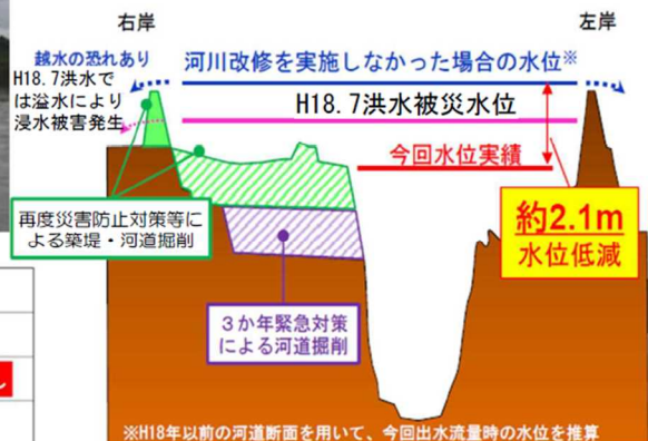
【羽月川堂崎地区 横断面図】
