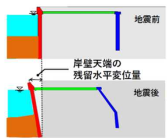
岸壁天端の変形イメージ
