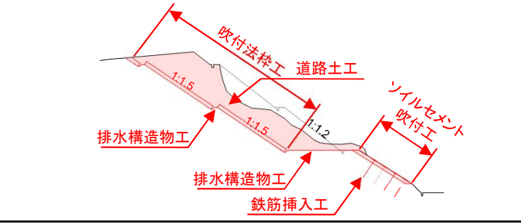
【断面図】A-A'断面
