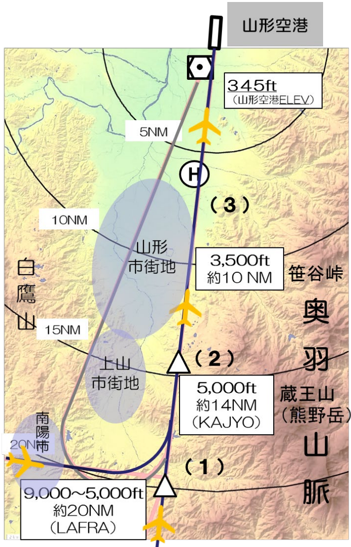
ILSにより進入するIFR機の経路
