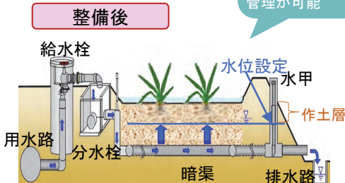
地下水水位制御システム (用水路と暗渠を接続することにより 地下からのかんがいも可能に)
