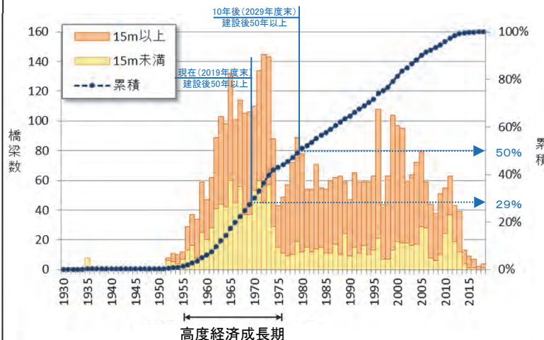
架設年次別の橋梁箇所数分布(北海道開発局管理) 出典:北海道開発局作成
