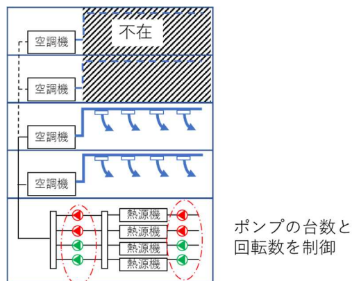
VVW 空調システム（変流量制御）
