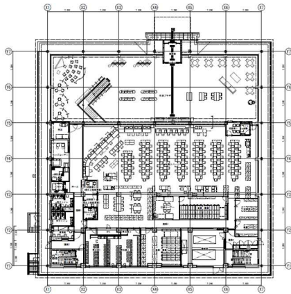
1階平面図
