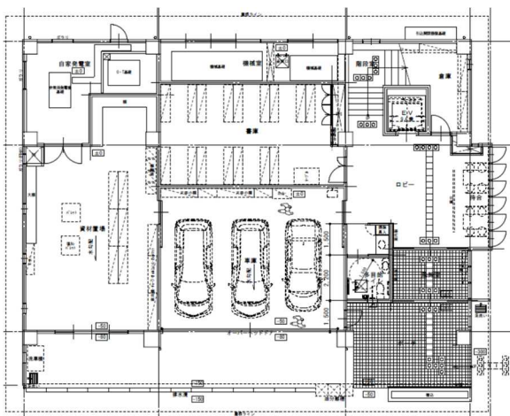
1階平面図
