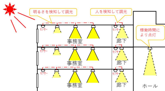
照明制御
