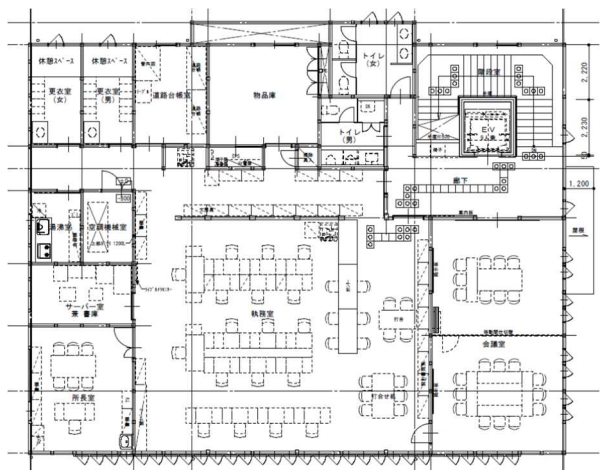
2階平面図
