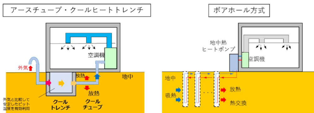
地中熱利用システム
