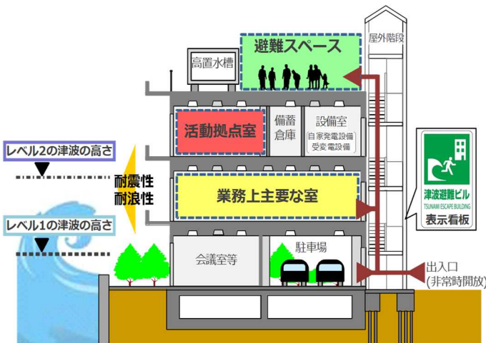
【官庁施設の津波対策（イメージ図）】
