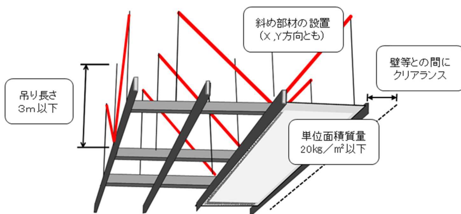
【官庁施設の天井耐震対策（イメージ図）】
