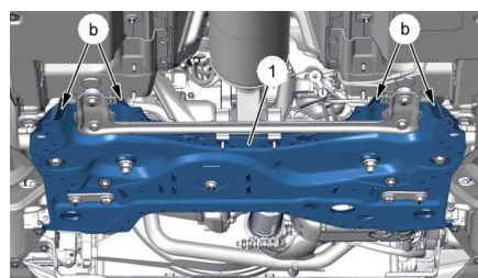
フロントサブフレーム
