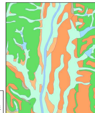
図2 地形分類図 (2万5千分1土地条件図)
