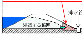
堤防の強化対策のイメージ
