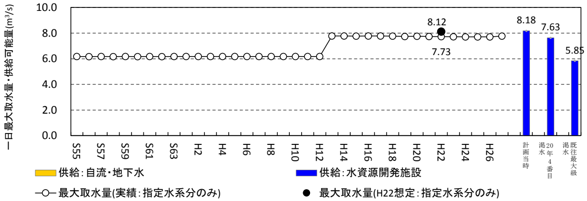
参考図表 6 4 都市用水 需要実績・想定と安定供給可能量の比較
