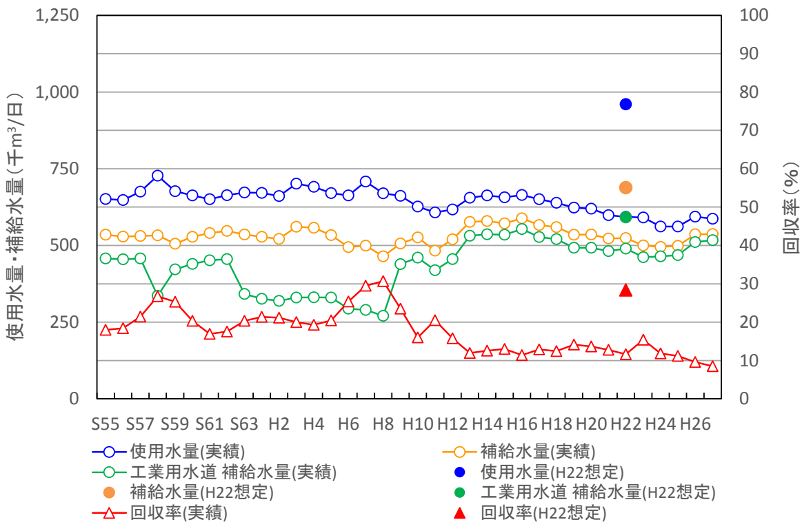
参考図表 4 4 工業用水使用水量, 補給水量, 工業用水道, 回収率の推移
