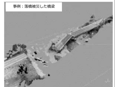
S f M (Structure from Motion) システムによる3Dデータモデルの作成
