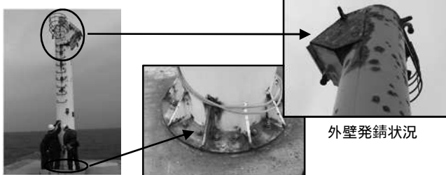
防波堤灯台
