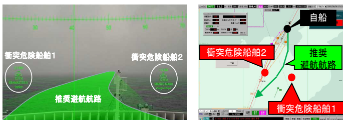
他船を回避する推奨避航航路の提示
