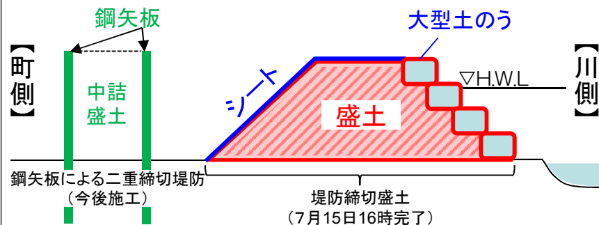
【緊急対策工事内容】 小田川左岸6k400
