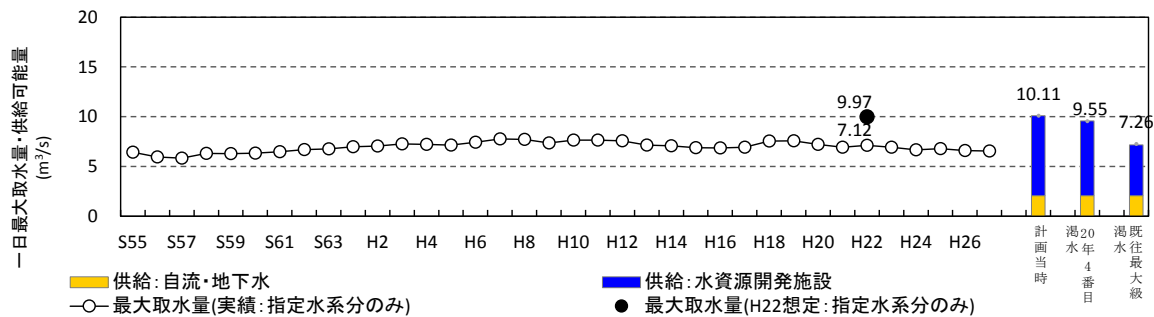
図 16 吉野川水系(指定水系依存)水道用水 需要実績・想定と安定供給可能量の比較
