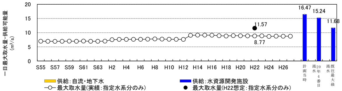
図 17 吉野川水系(指定水系依存)工業用水 需要実績・想定と安定供給可能量の比較
