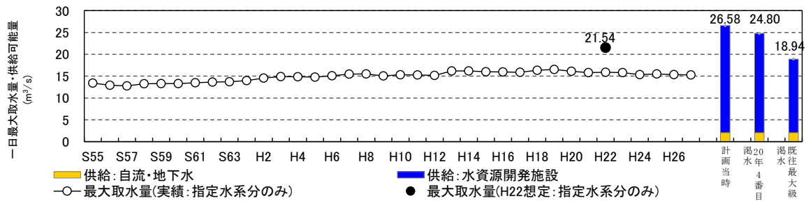
図 15 吉野川水系(指定水系依存)都市用水 需要実績・想定と安定供給可能量の比較
