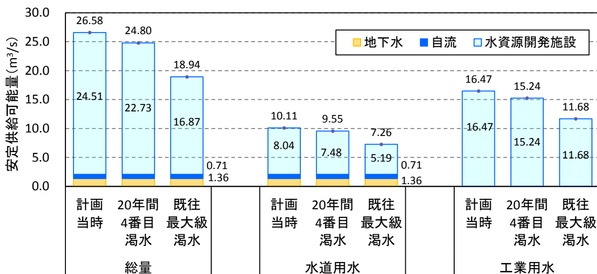
図14 吉野川水系 安定供給可能量
