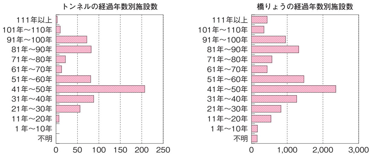
図表1-3-2-16 地域鉄道の施設の現状 (トンネル・橋りょうの経過年数) (2015年度末実績)
