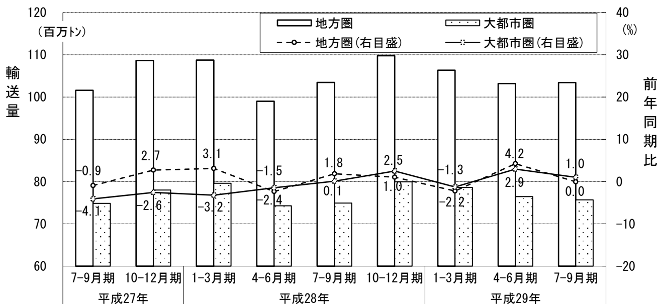
図 3-3-(2) 内航船舶輸送貨物量の推移(地方圏・大都市圏、平成27年7-9月期~29年7-9月期)
