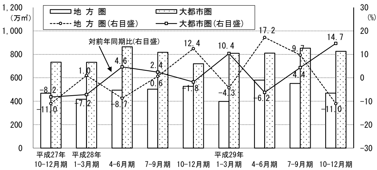
図 2-4-(2) 建築着工床面積(非居住用)の推移(地方圏・大都市圏、平成27年10-12月期~29年10-12月期)
