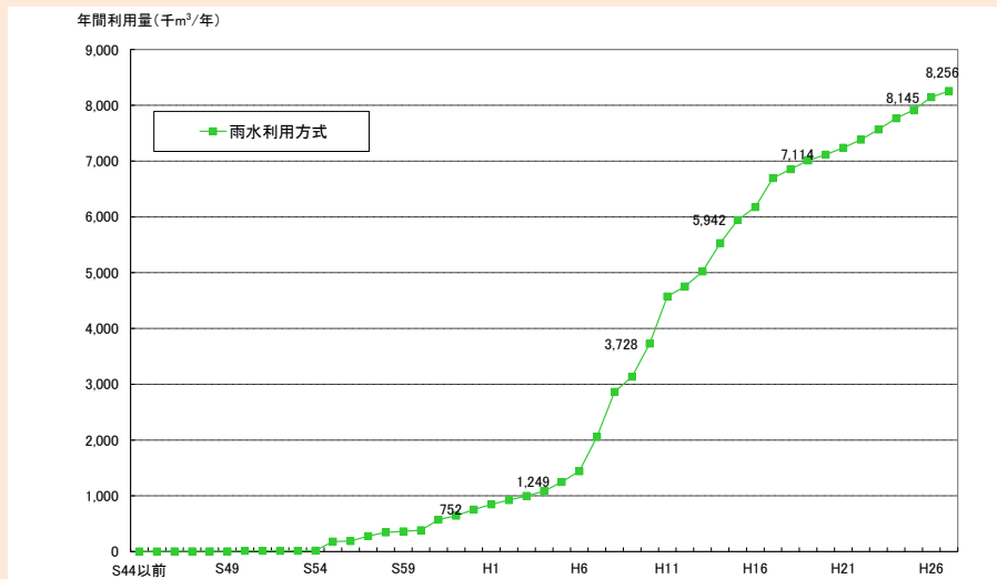
図3-2-4 雨水年間利用量の推移（雨水利用方式）
