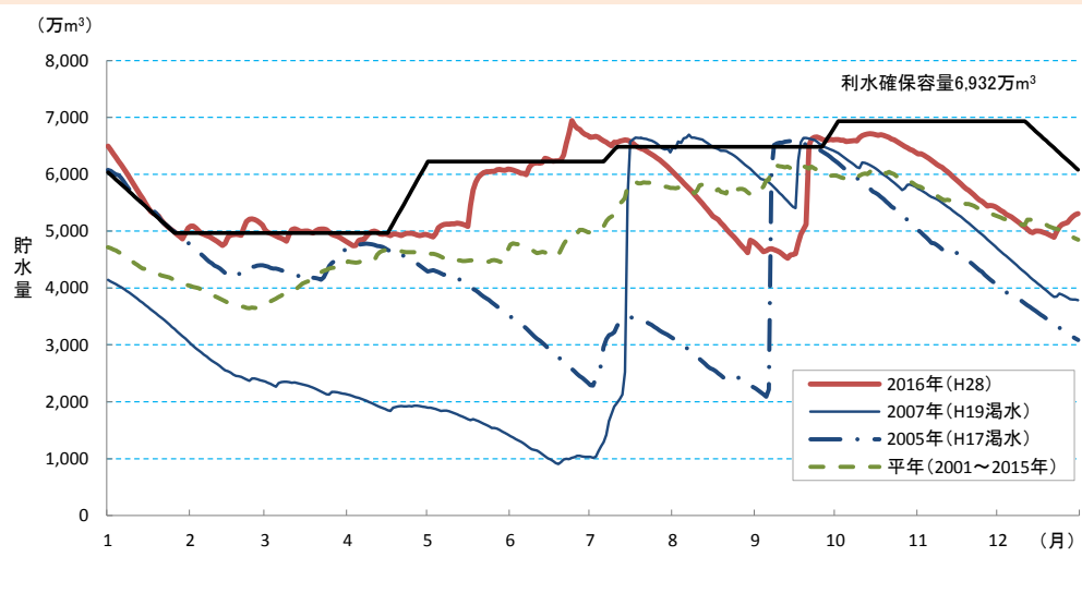
図3-7-15 銅山川3ダム（吉野川水系）貯水量図
