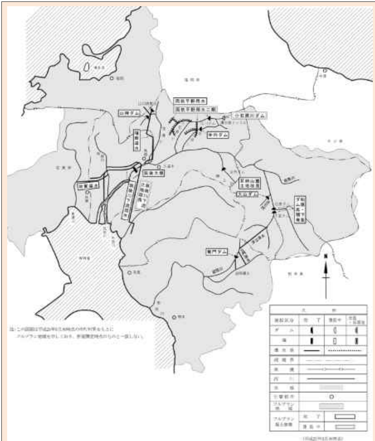
図3-1-11 筑後川水系における水資源開発事業の位置図
