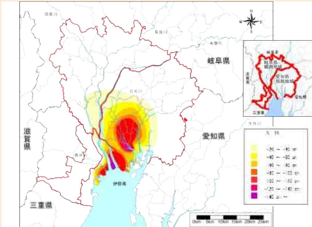
図 3-3-3 濃尾平野地盤沈下防止等対策要綱対象地域及び累積沈下量
