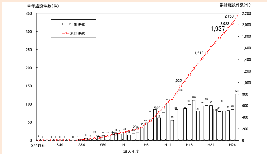
図3-2-3 雨水利用施設数の推移
