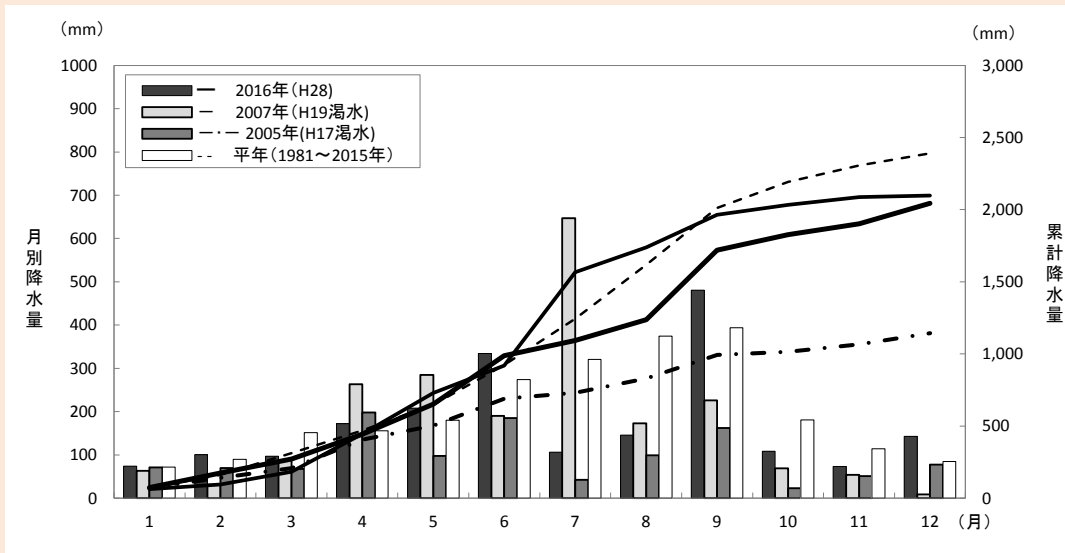
図3-7-14 降水の状況（新宮ダム上流域）
