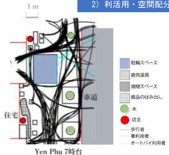
図2 ターミナル前面歩道占用とユーザー動線
