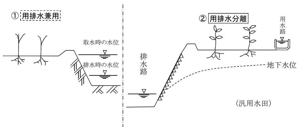
参考 2-4-2 用排水の分離による汎用水田化
