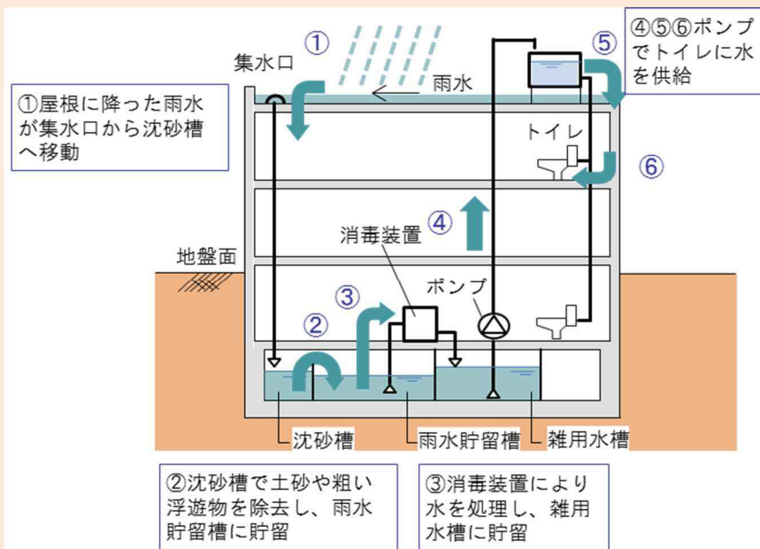
図4-2-7 雨水利用の事例 (熊本地方合同庁舎A棟 (熊本県) 配水系統図)
