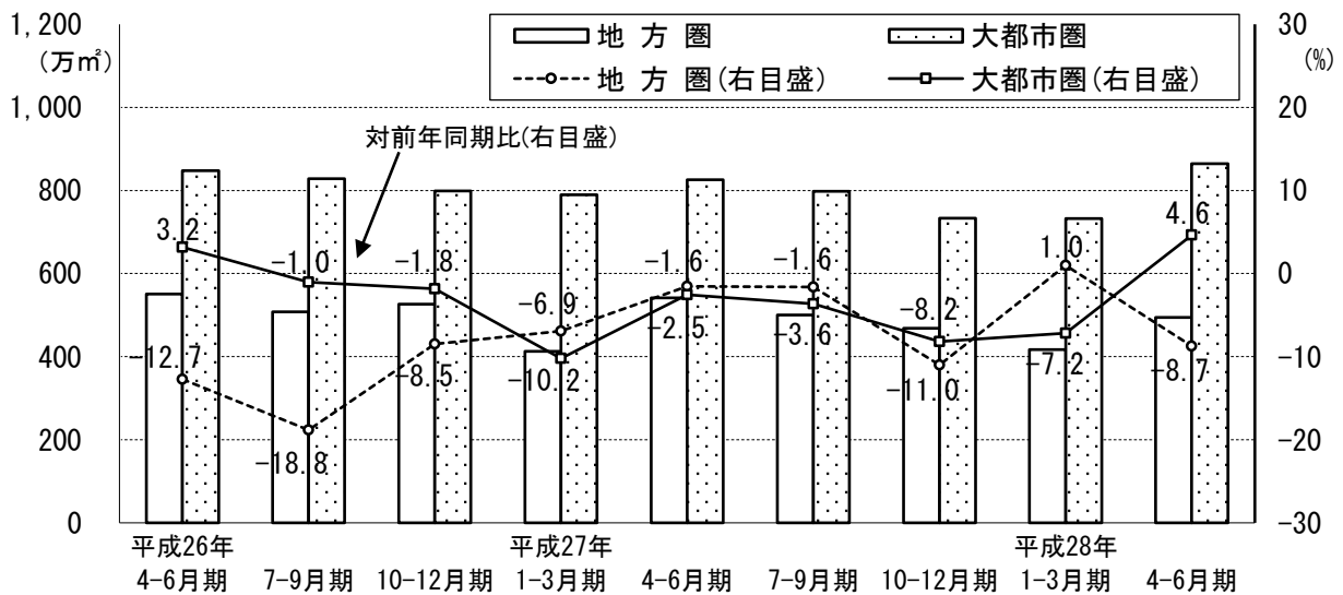
図 2-4-(2) 建築着工床面積(非居住用)の推移(地方圏・大都市圏、平成26年4-6月期~28年4-6月期)
