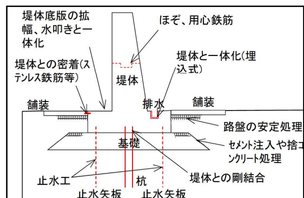
港湾における防潮堤(胸壁)の粘り強い構造の工夫【耐津波の例】
