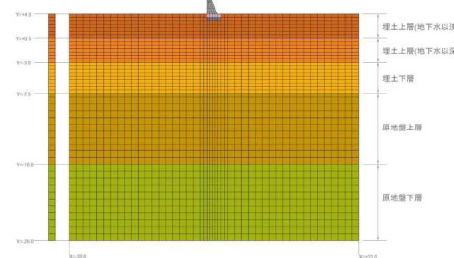
胸壁の動的FEM解析モデルのイメージ
