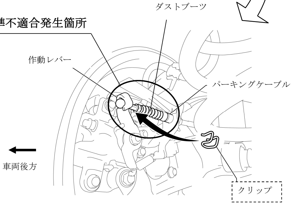
A 視：駐車ブレーキ 拡大図
