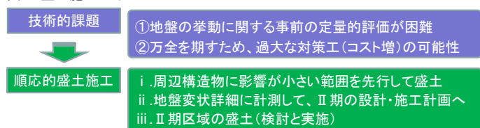
図3 盛土施工のイメージ
