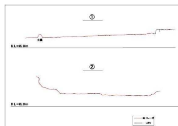
地上レーザーと三次元モデルを比較した断面図
