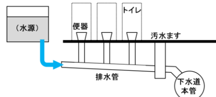
左：マンホールトイレ 右：マンホールトイレの概念図
