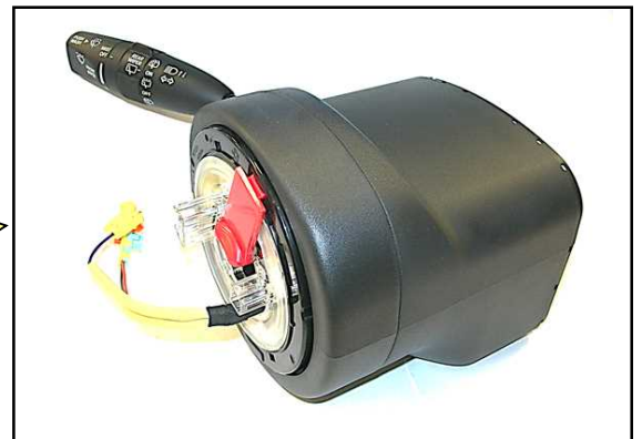
横滑り防止装置 ステアリング・コラム・コントロール・ユニットに内蔵
