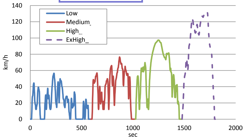
WLTC(Class3b)
