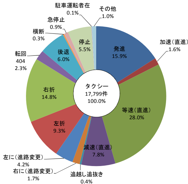
図 61 タクシーの行動類型別事故件数の割合（平成25年）
