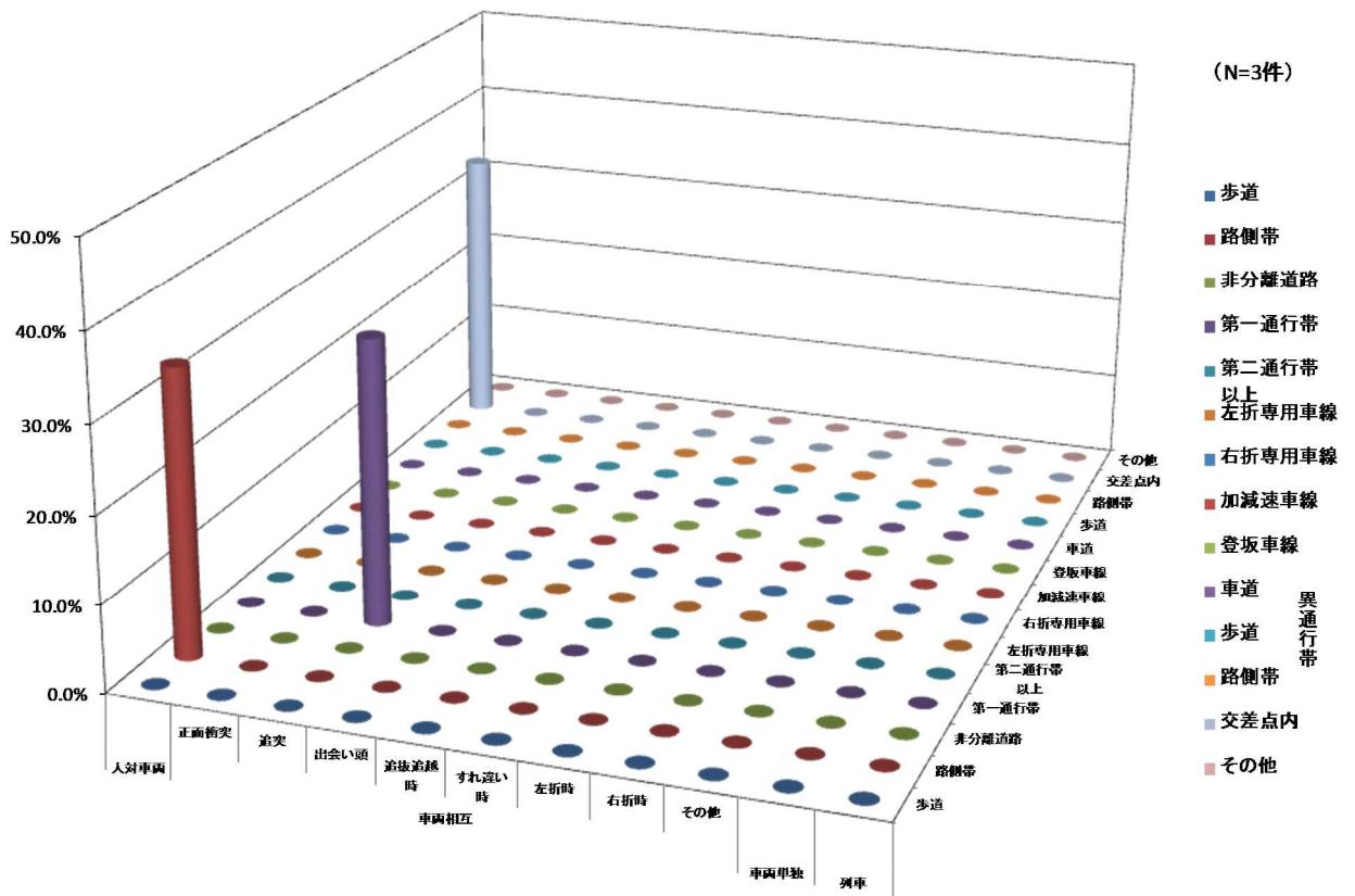
図 53 貸切バスの事故類型別、衝突地点別死亡事故件数の構成比（%）（平成25年）
