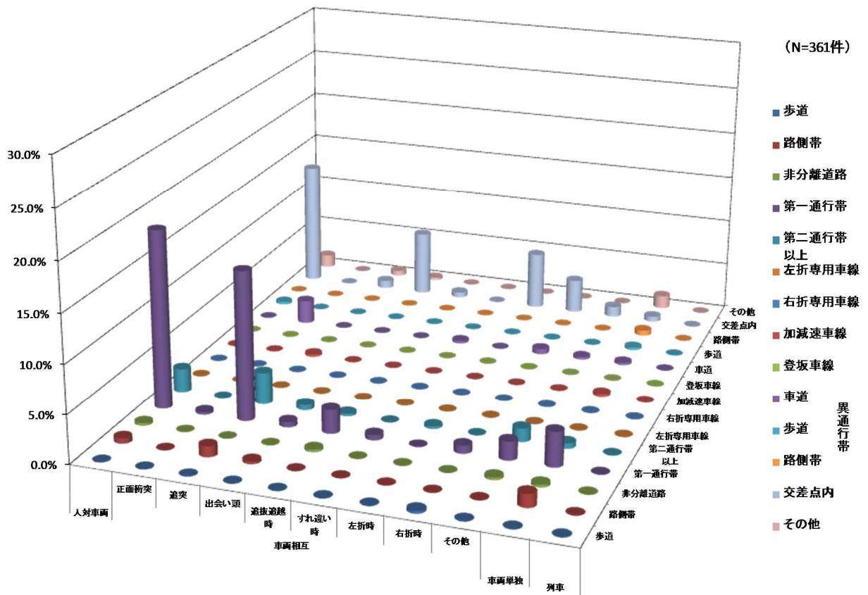
図 87 トラックの事故類型別、衝突地点別死亡事故件数の構成比（%）（平成 25 年）
