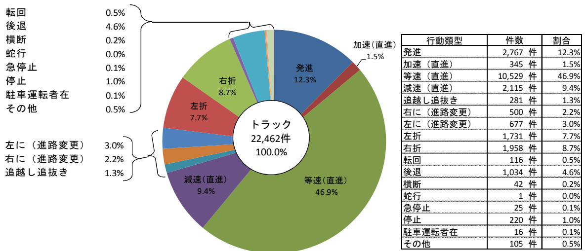
図 78 トラックの行動類型別事故件数の割合（平成25年）
