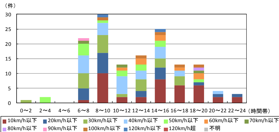
図58 貸切バスの追突の事故件数の危険認知速度別発生時間帯分布（件）（平成25年）
