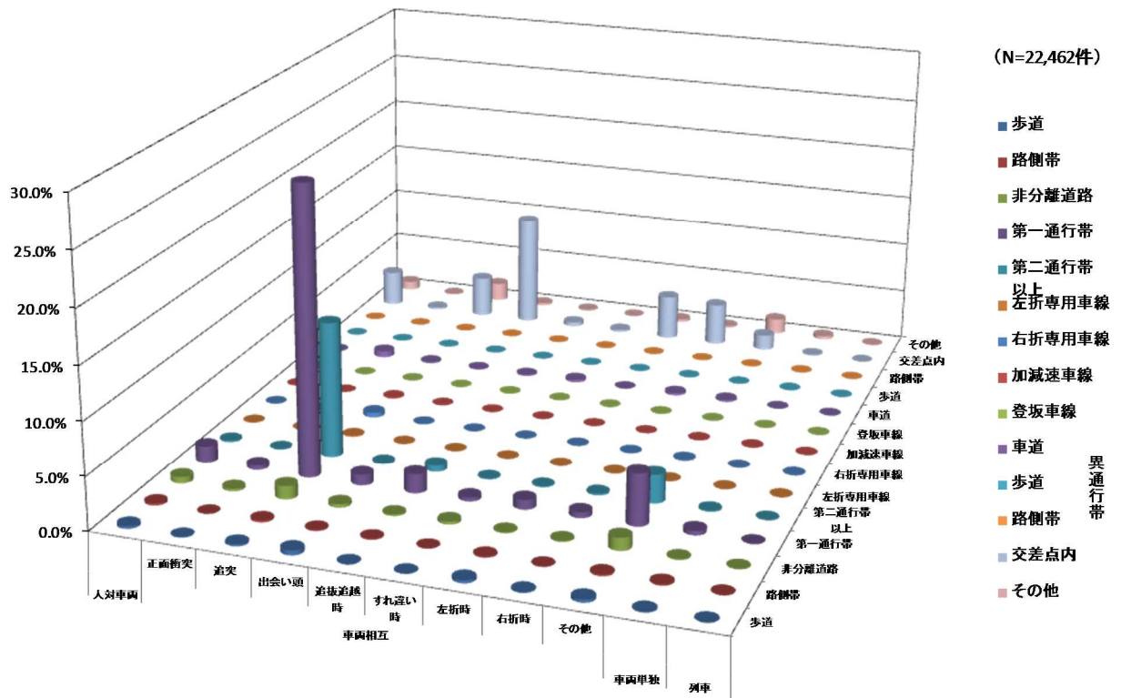
図 86 トラックの事故類型別、衝突地点別事故件数の構成比 (%) (平成 25 年)
