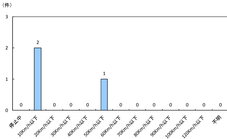
図 57 貸切バスの危険認知速度別の死亡事故件数（平成25年）
