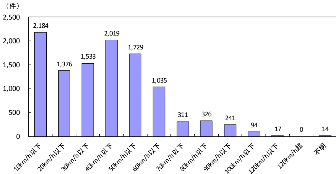
図 93 トラックの危険認知速度別の追突事故件数（平成25年）
