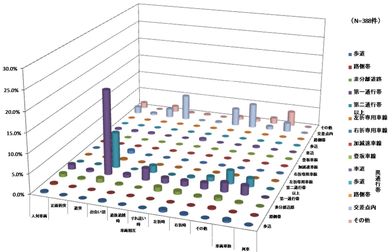
図 52 貸切バスの事故類型別、衝突地点別事故件数の構成比 (%) (平成25年)
