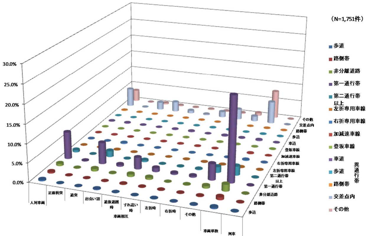
図 34 乗合バスの事故類型別、衝突地点別事故件数の構成比 (%) (平成25年)
