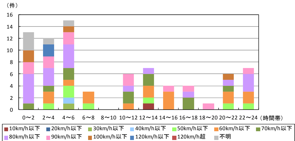
図 91 トラック追突の事故件数の危険認知速度別発生時間帯分布 (平成25年)
