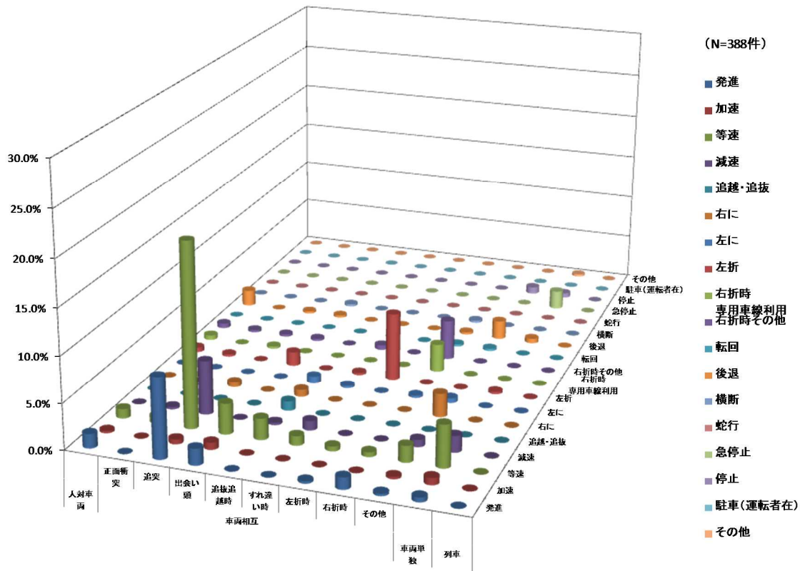
図 54 貸切バスの事故類型別、行動類型別事故件数の構成比（%）（平成 25 年）
