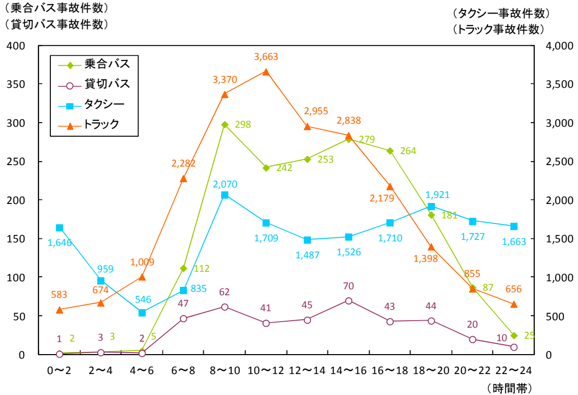
図 22 業態別時間帯別交通事故件数 (平成25年)
