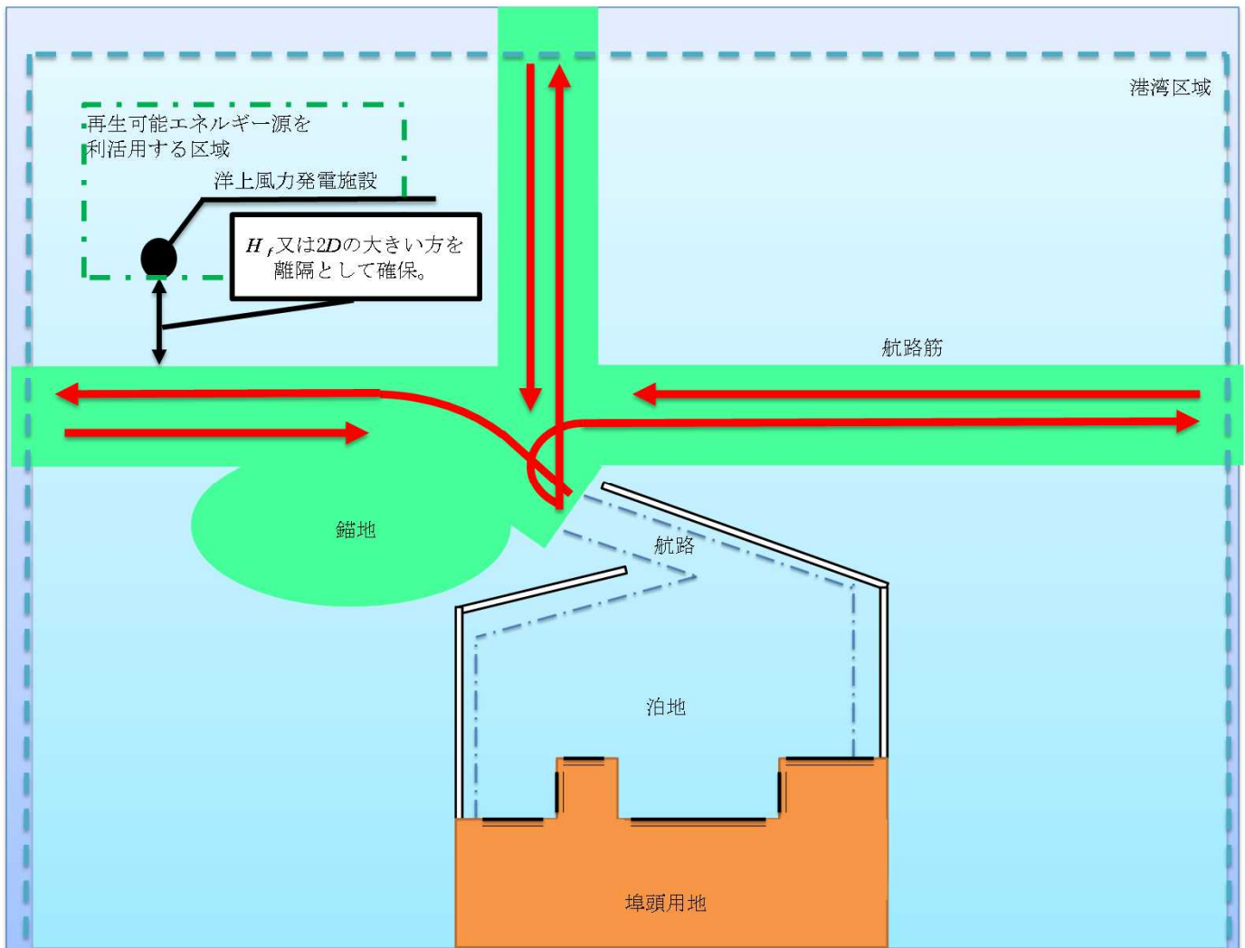
《 航路筋等との離隔の例 》
