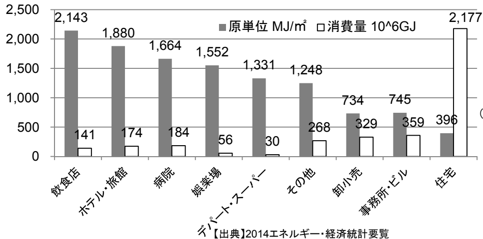
エネルギー消費量(新築フロー)【推計】
