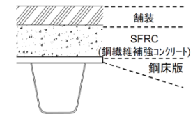
SFRC補強
