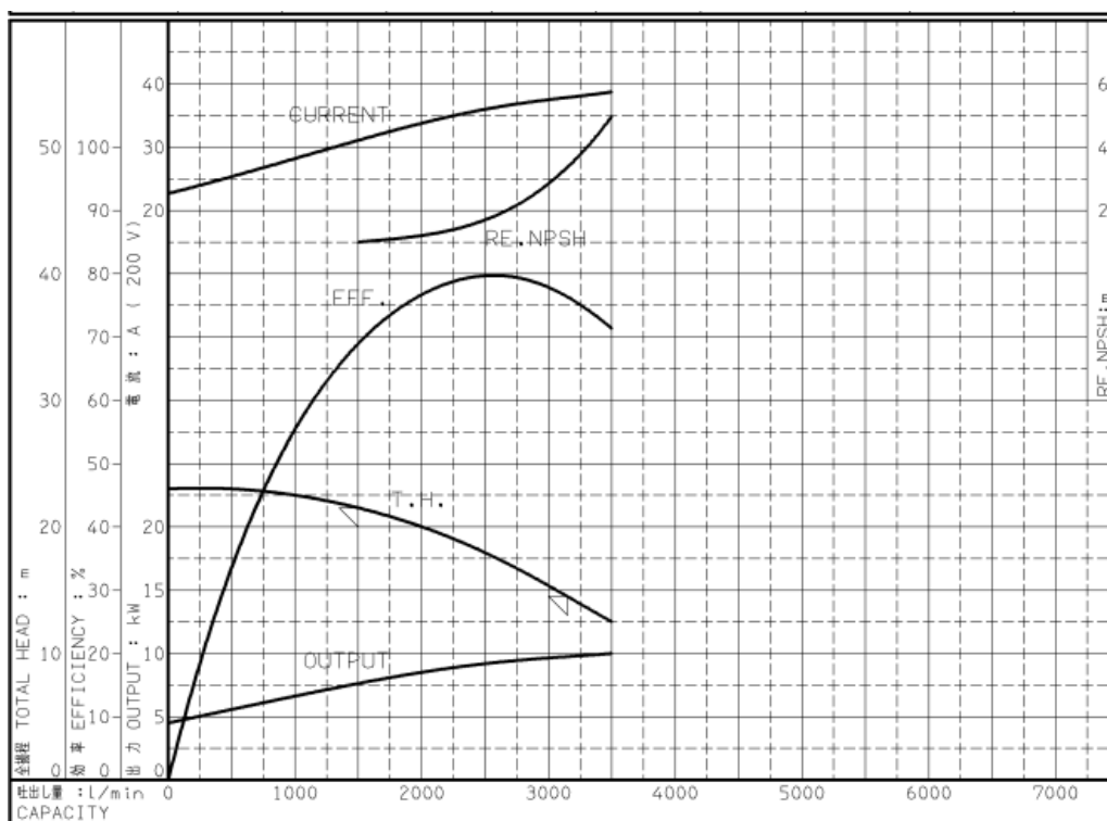
図 3.12 冷却水ポンプの P-Q 特性
