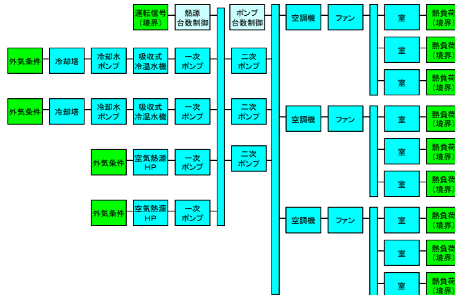
(4) 空調システム全体の構築例
