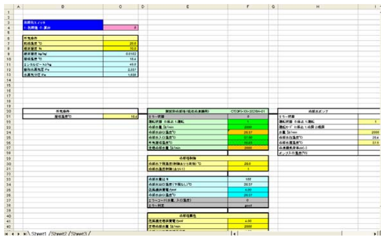
図 3.10 冷却塔オブジェクトの貼り付け完了
