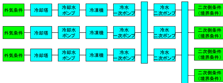
(3) 一次側サブシステムの構築例
