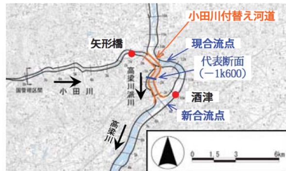
小田川付替事業の平面図
