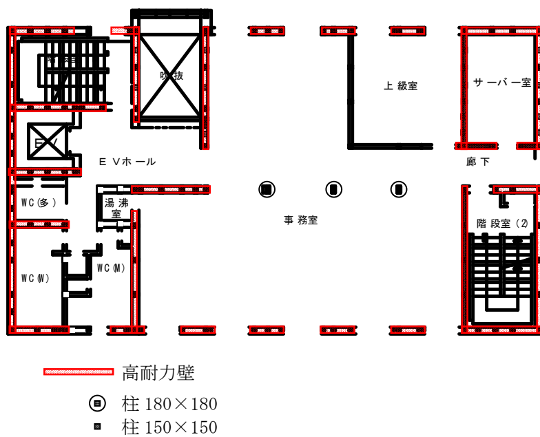
図 2.3-6 3階 耐力壁及び柱の配置
