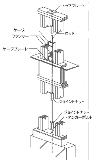
図 2.3-21 タイダウン金物 (~280kN 程度)
