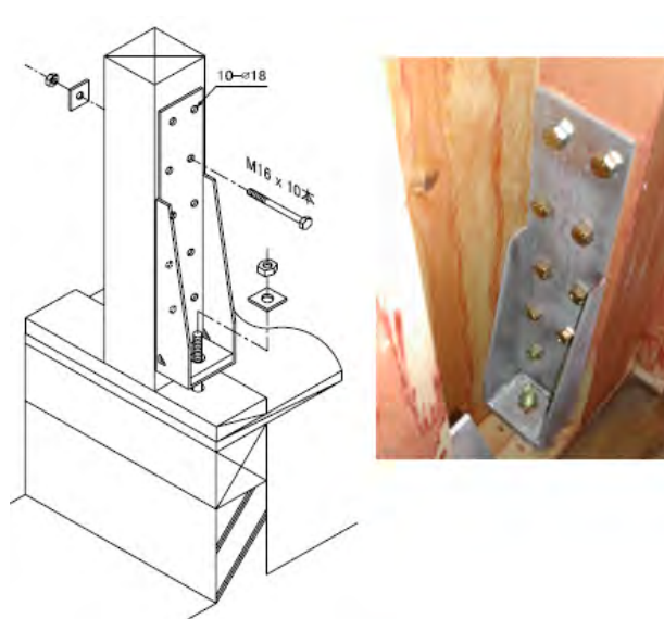
図 2.3-23 HD 金物例 (100kN 級)
