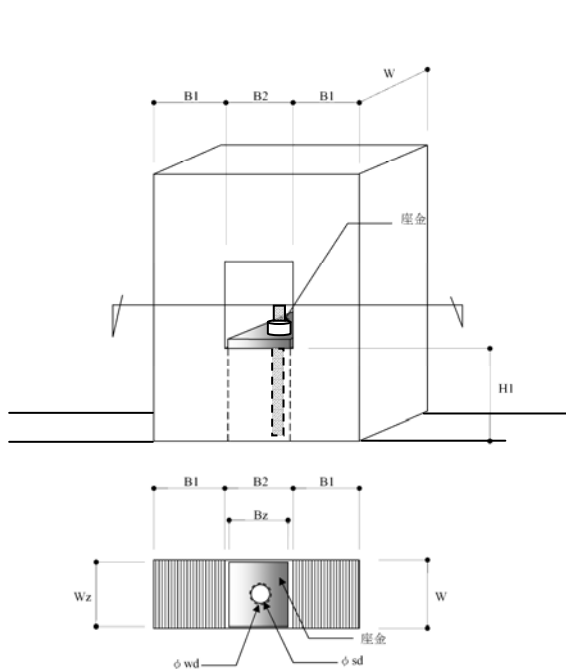
図 2.3-20 引きボルト接合例(100kN 超)
