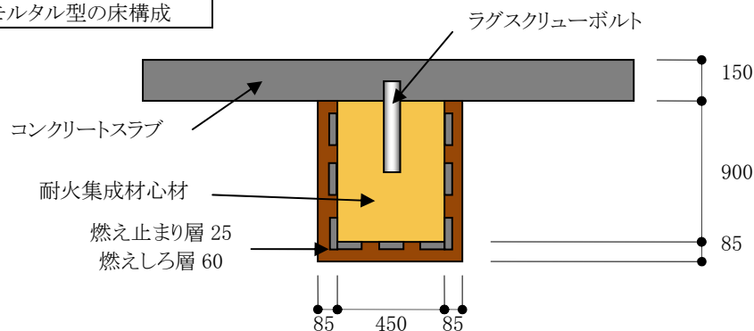
図 2.3-11 床（モルタル型）の仮定断面
